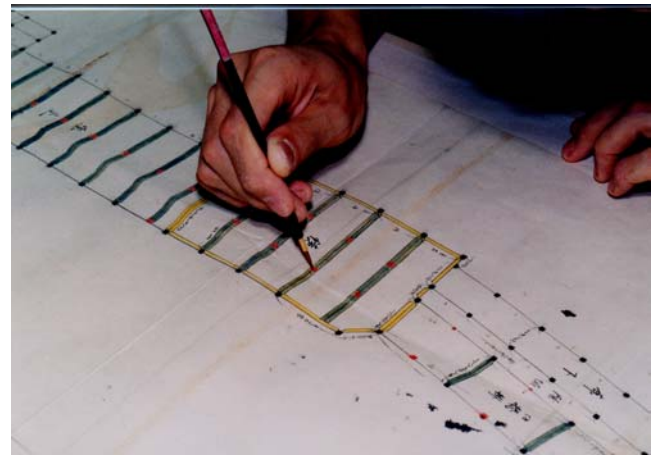
図16 剥落止め
